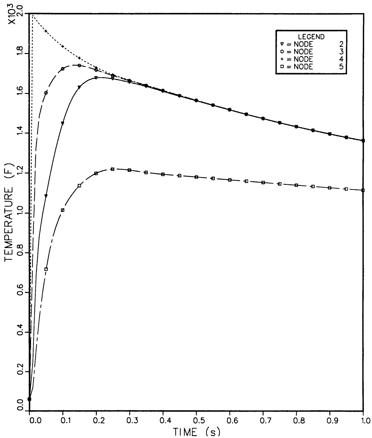
Fig. 17. Temperatures.
