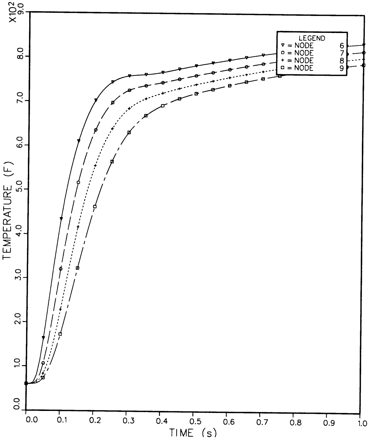
Fig. 18. Temperatures.
